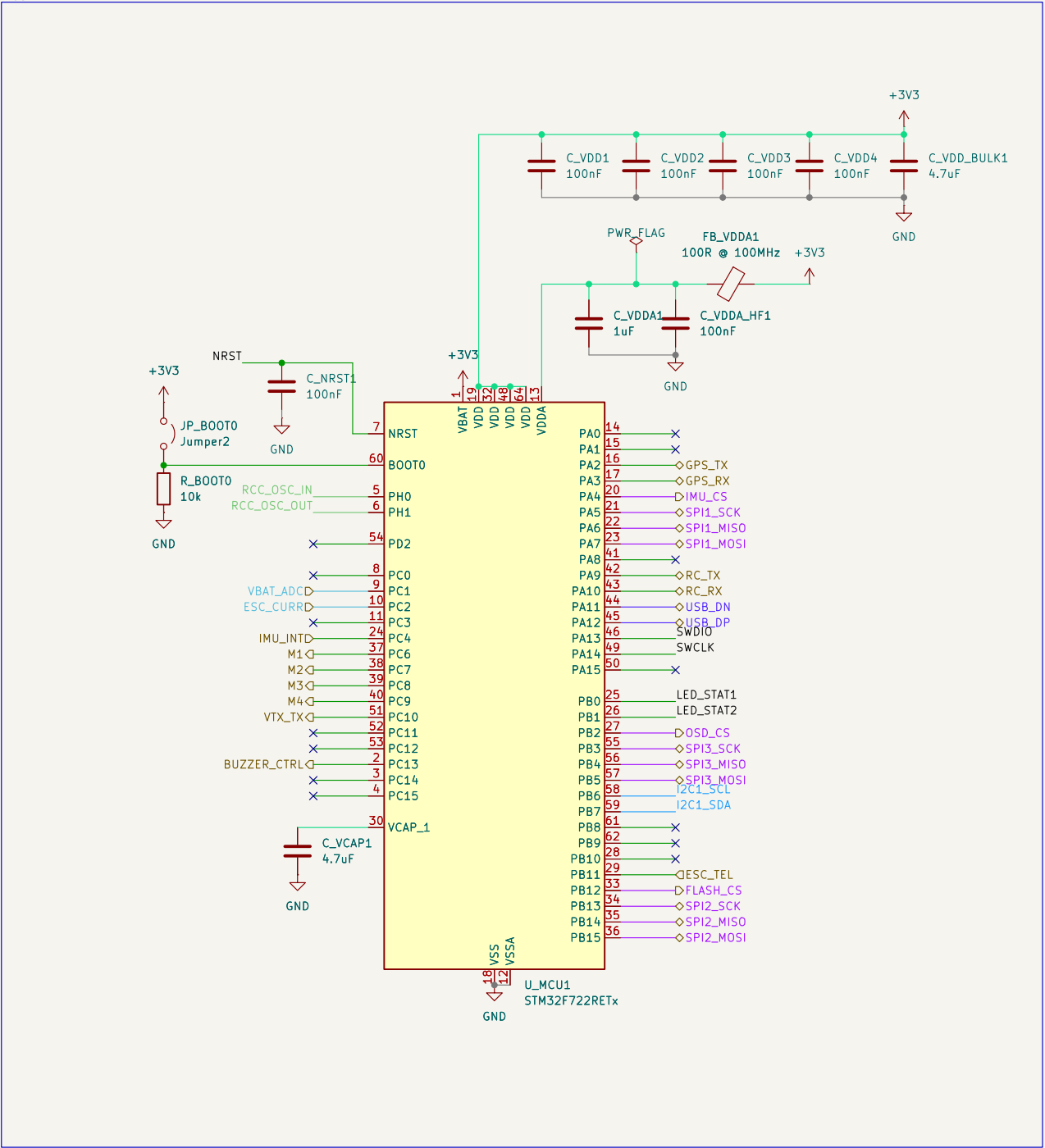
MCU
