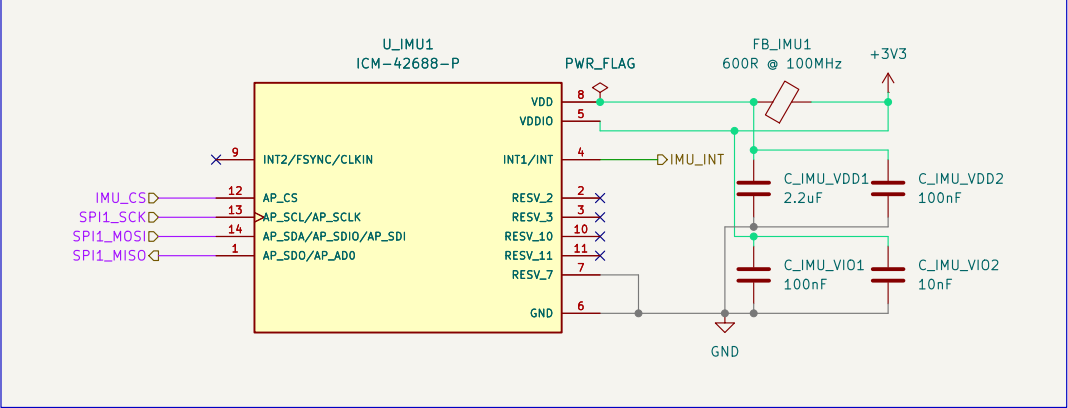
IMU (żyroskop)
