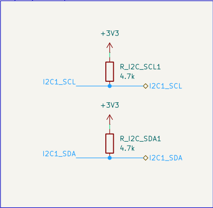
Rezystory Pull-Up do I2C1
