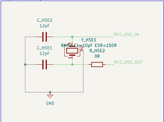
Oscylator kwarcowy
