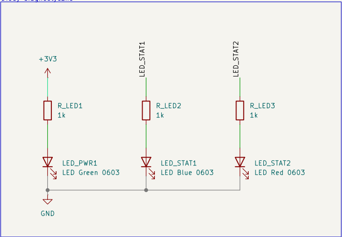
Diody diagnostyczne
